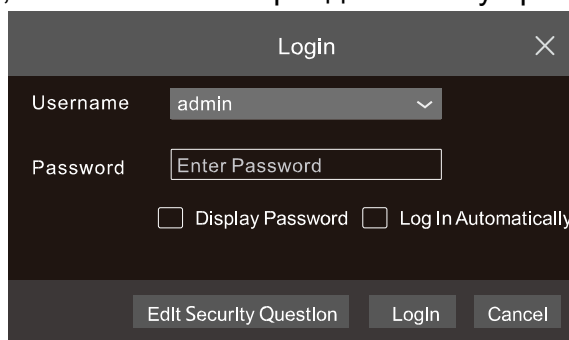
Рис. 1.2. Окно авторизации
